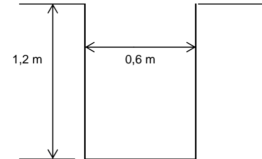
Grabenprofil Wasser:
