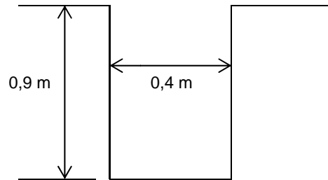
Grabenprofil Strom:
