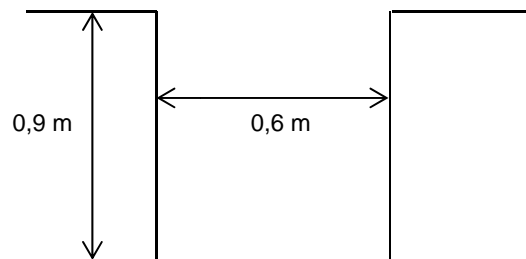
Grabenprofil Gas und Strom:
